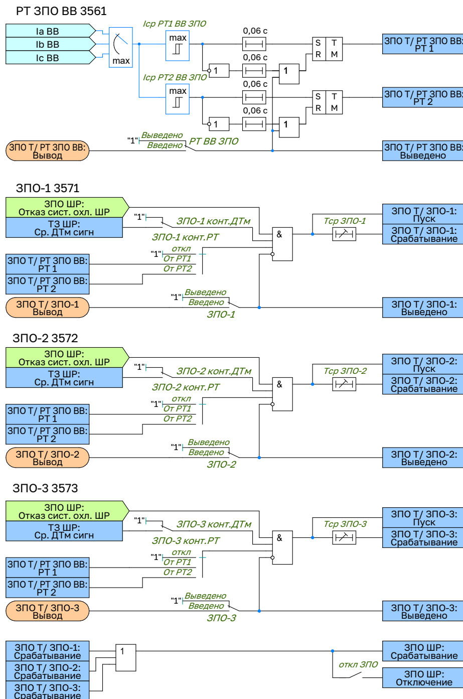
Рисунок 2.20 – Функциональная схема логики ЗПО
